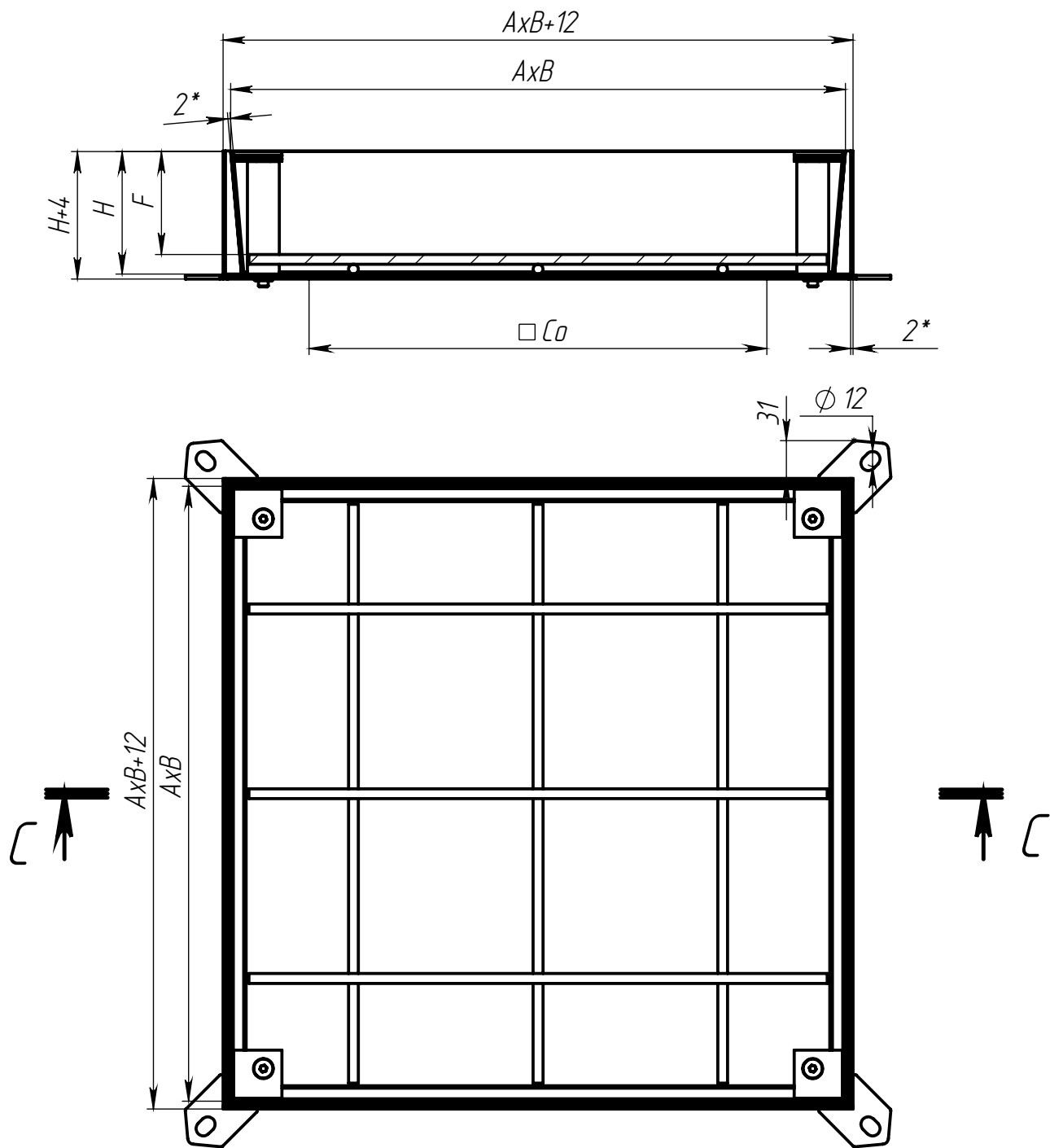
СЕЧЕНИЕ С-С (1 : 5)
